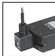
TYPE 04: PV Epoxy encapsulated EN/IEC 60079-18
