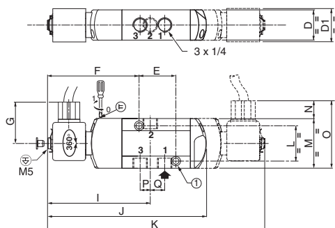
TYPE 05: WBLP Metal cap/PBT EN/IEC 60079-7, EN/IEC 60079-18 and EN/IEC 60079-31
