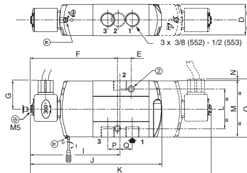
TYPE 06: WBLP Metal cap/PBT EN/IEC 60079-7, EN/IEC 60079-18 and EN/IEC 60079-31
