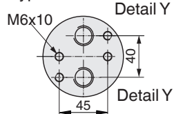
Type 5000U
