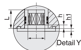
Type 5000U
