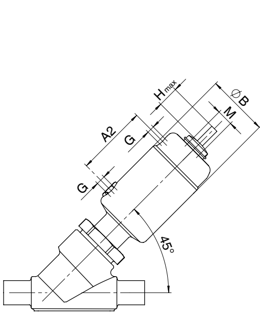
Actuator size 0, 1
