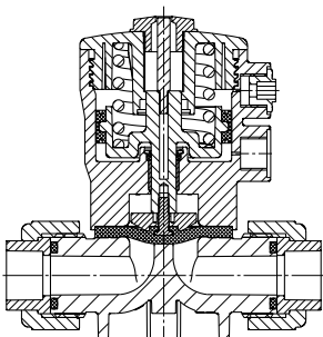
GEMÜ 630
