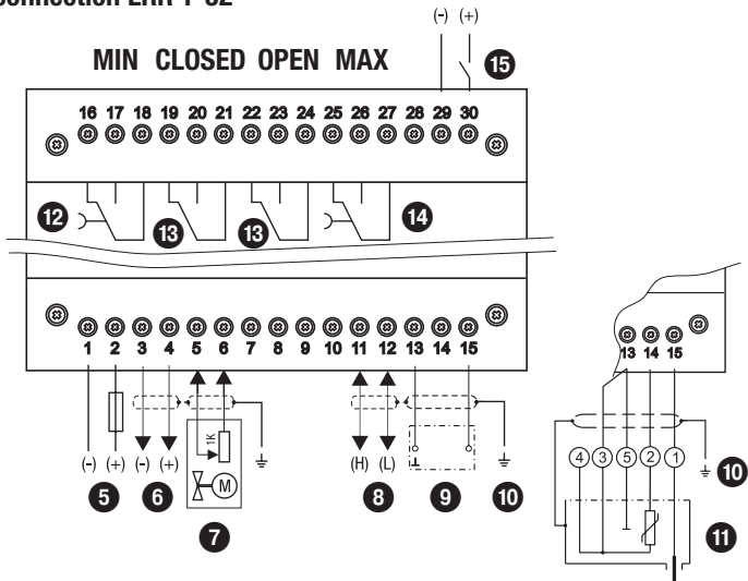
Fig. 1 LRR 1-52, LRR 1-53
