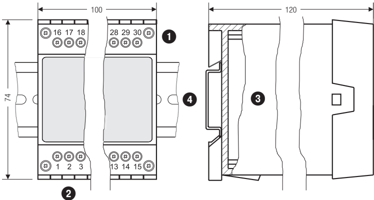
Fig. 1 LRR 1-52, LRR 1-53
