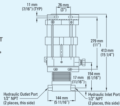
ATV-8 pumps
