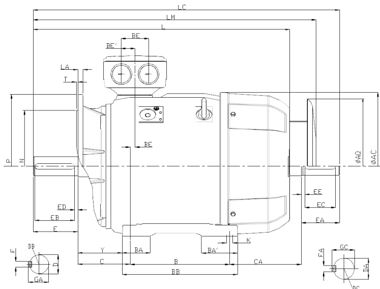
Fuß- Flanschbauformen feet / flange type of construction
