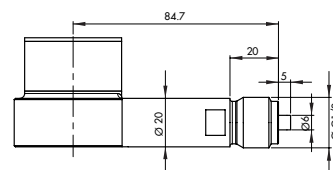
Radialer Gasanschluss connexion de gaz radiale radial gas connection
